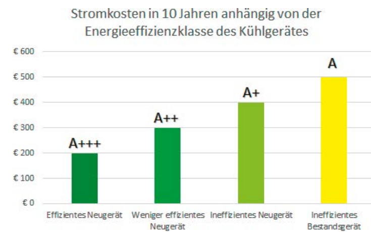
Kühlschrank mit 130 l Kühlinhalt und Tiefkühlfach, Strompreis von 20 Cent/kWh
