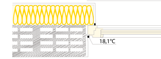
Abb. 22 | Falsch: Fenster und Dämmebene weisen eine Lücke auf, Richtig: Überdämmter Fensterstock
